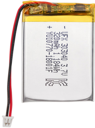
Model: UFX 303040 320mAh 3.7V
