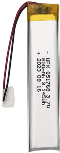
Model: UFX 851768 850mAh 3.7V
